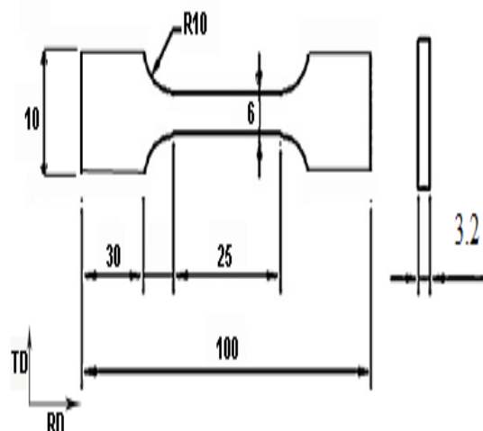
شکل (۲) طرح کلی آزمون کشش طبق استاندارد ASTM E8 (M).
