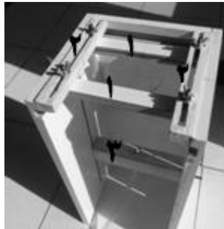
شکل (۶) دستگاه سیستم کنترل موقعیت
