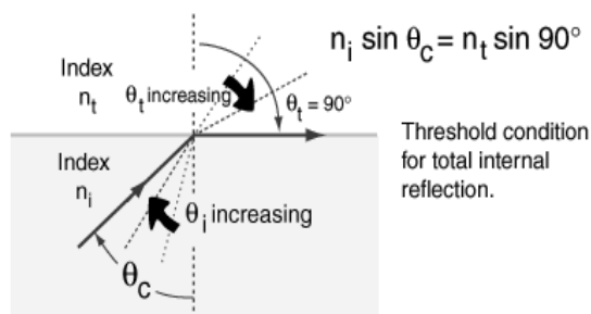
شکل (۲): نتیجه برابری زاویه تابش با زاویه حد
