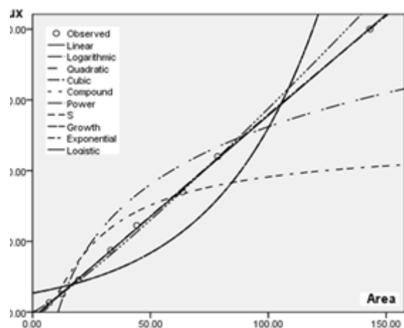
شکل (۹) نمودار لوکس بر حسب مساحت عدسی - بر اساس مدل
