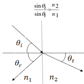
شکل (۱): نمایش عبور و بازتاب پرتو نور در مرز دو محیط شفاف
