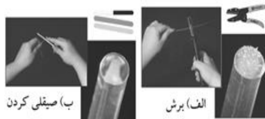
شکل (۵): آماده سازی فیبرها
