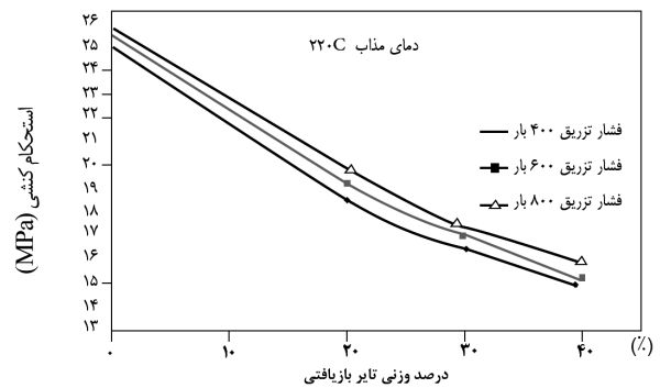
شکل (۴) تأثیر درصد وزنی پودر تایر بازیافتی بر روی استحکام کششی کوپلیمر با دمای مذاب ۲۲۰ °C.
